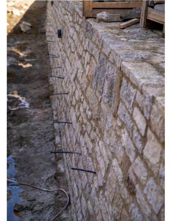
Mauerwerkssanierung Leinekanal Göttingen: Homogenisierung der Bestandswand durch Injektion.
